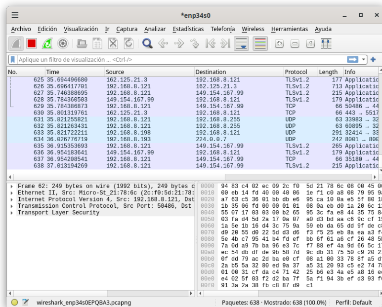
FIGURA 19.2: wireshark: interfaz de captura por defecto
